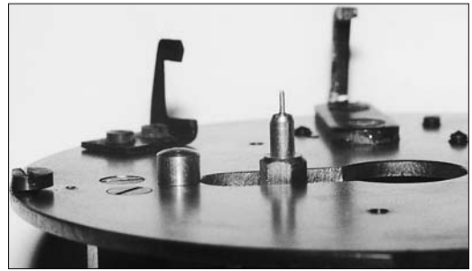
Abb. 10 A: Schreibstift der Wächteruhr mit Rüttelschreiber »Vibrograph«.
