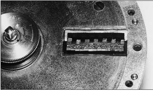
Abb. 8: Papierscheiben-Wächteruhr mit Zahlenmarkierung für 12 Kontrollstellen und zusätzlichem Kontrollzeichen »A«.
