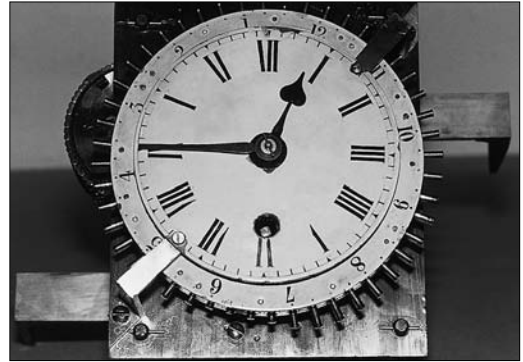
Abb. 3: Englische Tisch-Wächteruhr um 1840 von Thwaites & Reed, London. Die Metallstifte werden durch Drücken eines Knopfes betätigt. Ein Exzenter drückt die Stifte kurz vor Beendigung des Zifferblattumlaufs wieder nach außen
