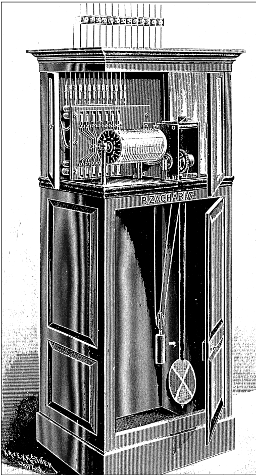
Abb. 12: Stationäre Wächter-Kontrolluhr von Zachariä, Leipzig. Von Elektromagneten betätigte Stahlstifte perforieren die Diagrammscheibe.
