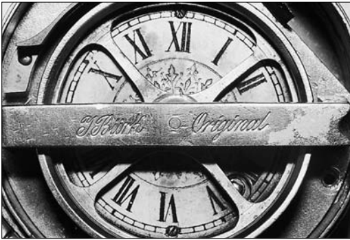
Abb. 6: Trommel-Wächteruhr Bürk-Original nach dem Patent von 1855. Zum Auswechseln des Papierstreifens muß der Bügel hochgeklappt und die Papiertrommel herausgenommen werden. Ab ca. 1930 wurde die Trommel durch einen Rändelknopf fixiert. Dieses Modell wurde bis in die 1960er Jahre hergestellt.
