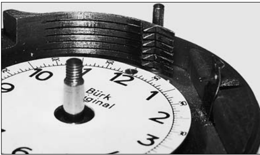
Abb. 7: Trommel-Wächteruhr Bürk Original, spätere Ausführung ohne Befestigungsbügel. Man erkennt die 6 Markierfedern mit Perforationspitzen sowie rechts die Markierspitze, die das Öffnen des Gehäuses registriert.
